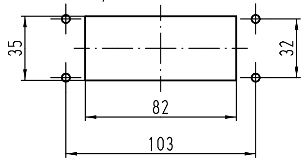
1:2 Montageausschnitt panel cut out
